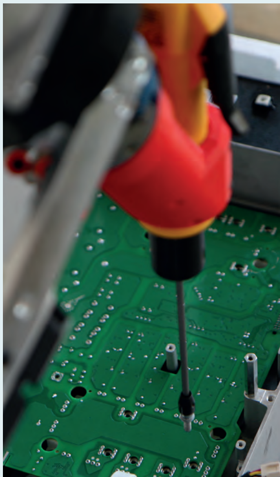
Teknologisk Institut har udviklet en robotløsning, som via visionsteknologi selv kan lokalisere skruehullerne på et emne og herefter skrue skrueene i. Foto: Teknologisk Institut
